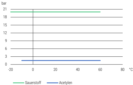
Druck-Temperatur-Diagramm pressure-temperature-diagram
