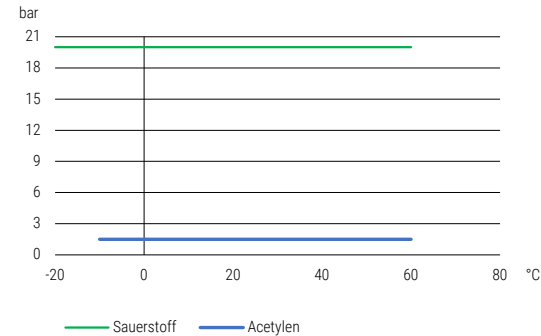
Druck-Temperatur-Diagramm pressure-temperature-diagram
