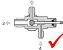
Rys. C: Częściowe otwarcie (5,5 obrotu w prawo od stanu całkowicie otwartego). Przyłącza 2, 3, 4 całkowicie otwarte.
