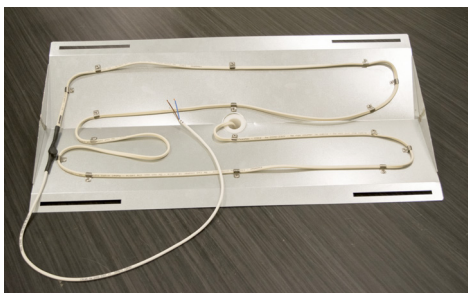
3. Lägg i värmekabeln och fäst i förmonterade fästen
