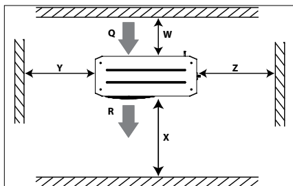
Bild 1: Minimum monteringsavstånd
