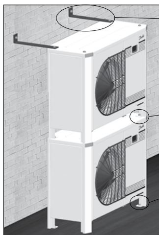
Obrázek 2: Montáž nad sebe
