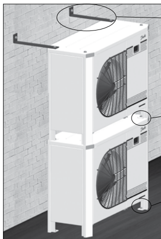
Bild 2: Staplingsmontering
