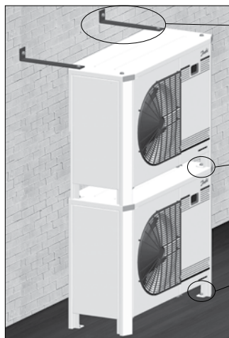
Imagem 2 : Montagem em pilha
