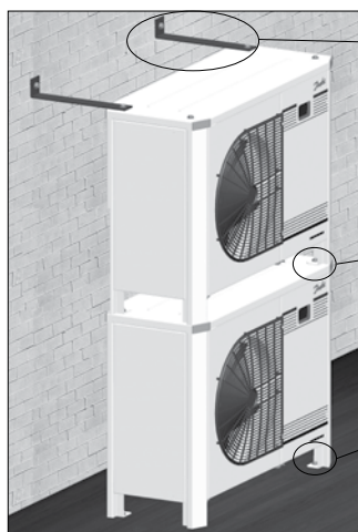
Рисунок 2: Многоуровневое размещение
