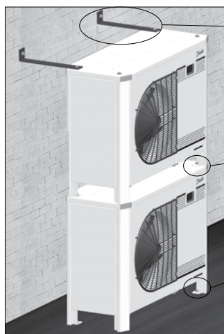
Illustration 2 : Montage superposé
