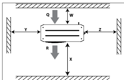
Bild 1: Mindestmontageabstände
