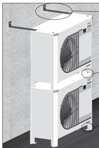
Rysunek 2: Montaż spiętrzony
