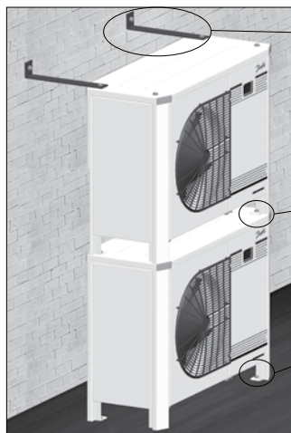
Ilustración 2: Montaje apilado
