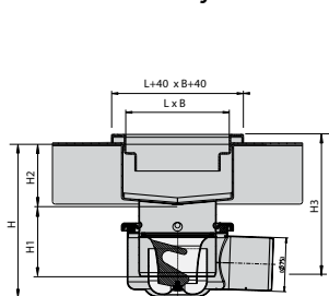
Spärrbrunn med vattenlås och sidoansluten underdel
