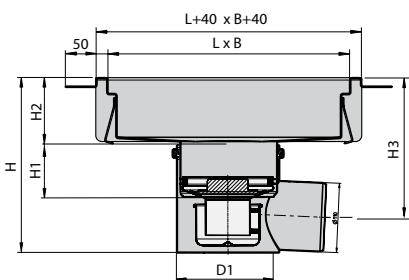
Köksbrunn med vattenlås och sidoansluten underdel
